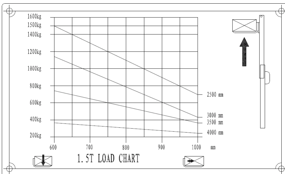
Диаграмма грузоподъёмности для 1,5 т
