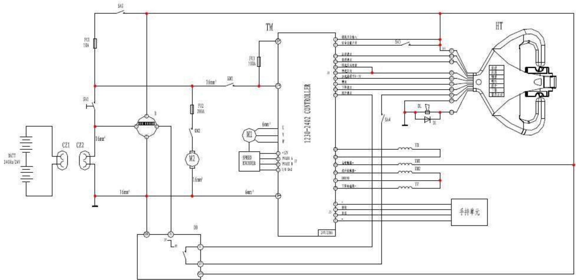
1230 Электрический штабелёр
