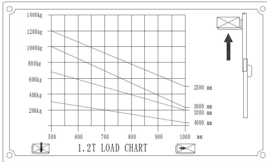
Диаграмма грузоподъёмности для 1,2 т
