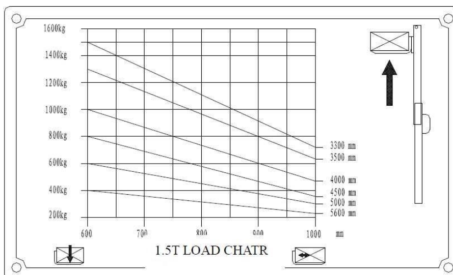
Диаграмма грузоподъёмности для 1,5 т
