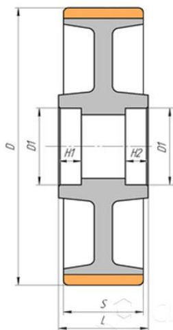
Схема опорного колеса для малой складской техники
