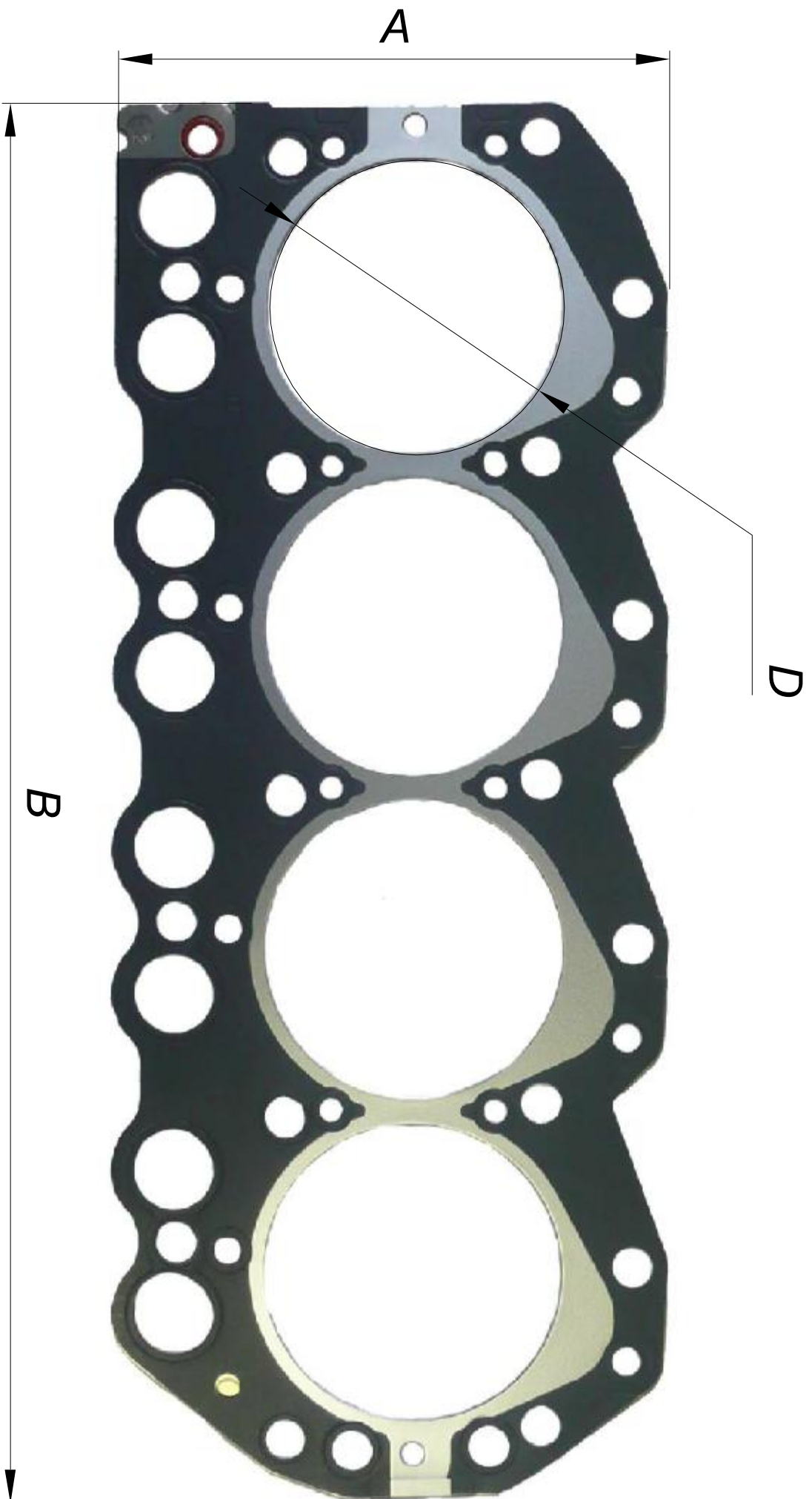
S-Толщина прокладки (для дизельных двигателей)
