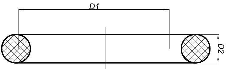
Тип 1 (см. О-кольцо)
